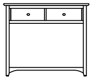
CONSOLE TABLE 2 DRAWER H: 770 W: 845 D: 350
