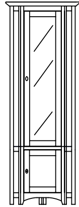
CORNER DISPLAY CABINET H: 1800 W: 650 D: 432
