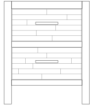
2 DRAWER BEDSIDE H: 550 W: 460 D: 420
