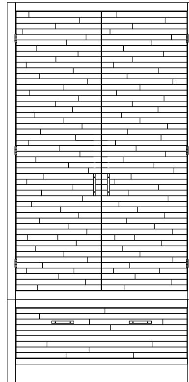
1 DRAWER WARDROBE H: 750 W: 2000 D: 1000
