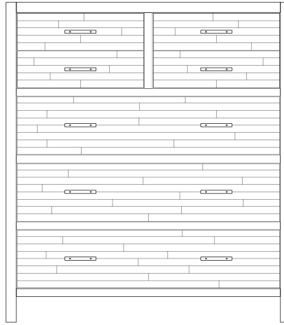
2 + 2 + 3 CHEST H: 1240 W: 1100 D: 450
